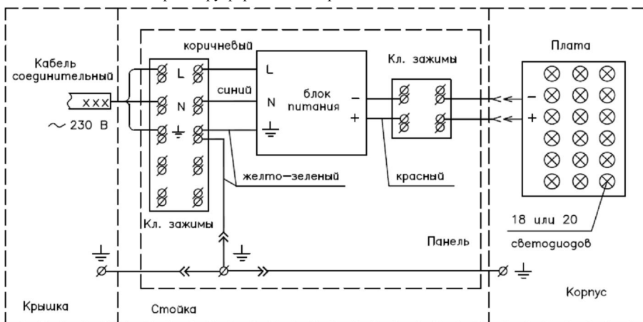
Рисунок 1. Схема электромонтажная светильника серии «Базз».
