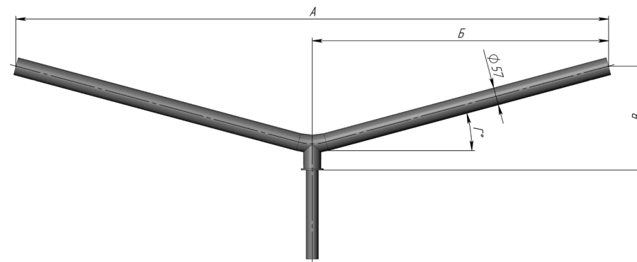
Рисунок 2. Габаритные и присоединительные размеры кронштейнов исполнений: SA-8-0,5-15, SA-8-1,0-15
