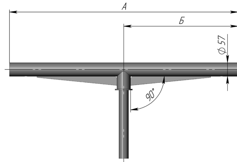
Рисунок 1. Габаритные и присоединительные размеры кронштейнов исполнений: SA-8-0,5, SA-8-1,0
